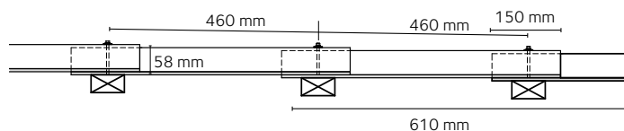
Længdesnit
