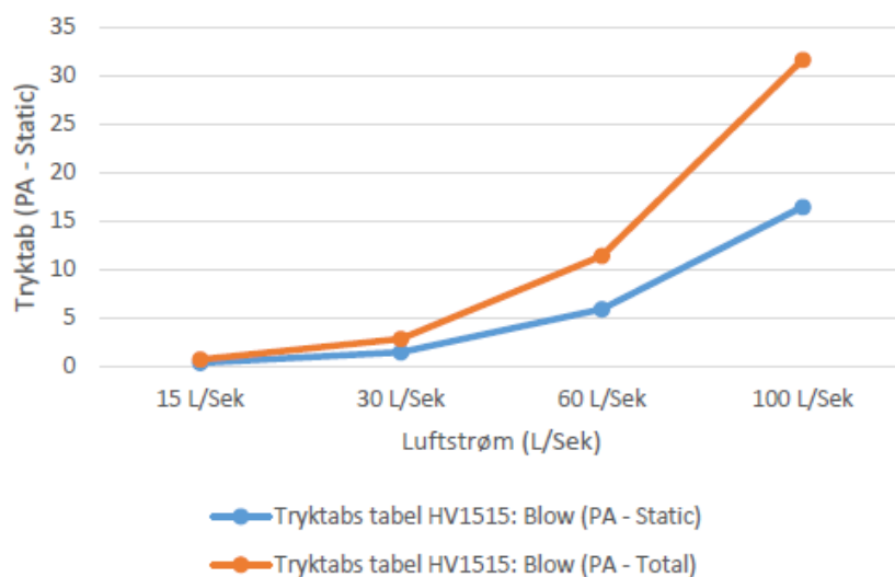
Tryktab HV15x15 med rundt ISO-rør (Luft ud)
